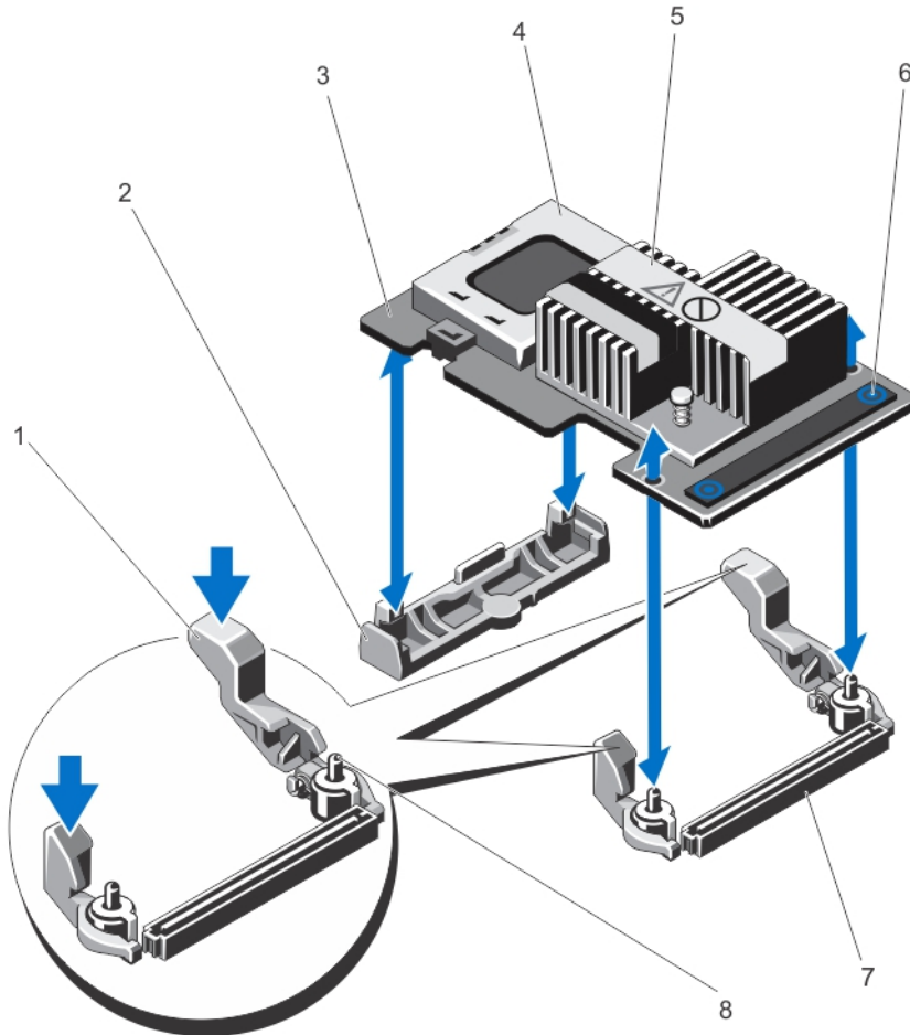
그림 3. PERC 미니 모놀리식 컨트롤러 분리 및 설치
